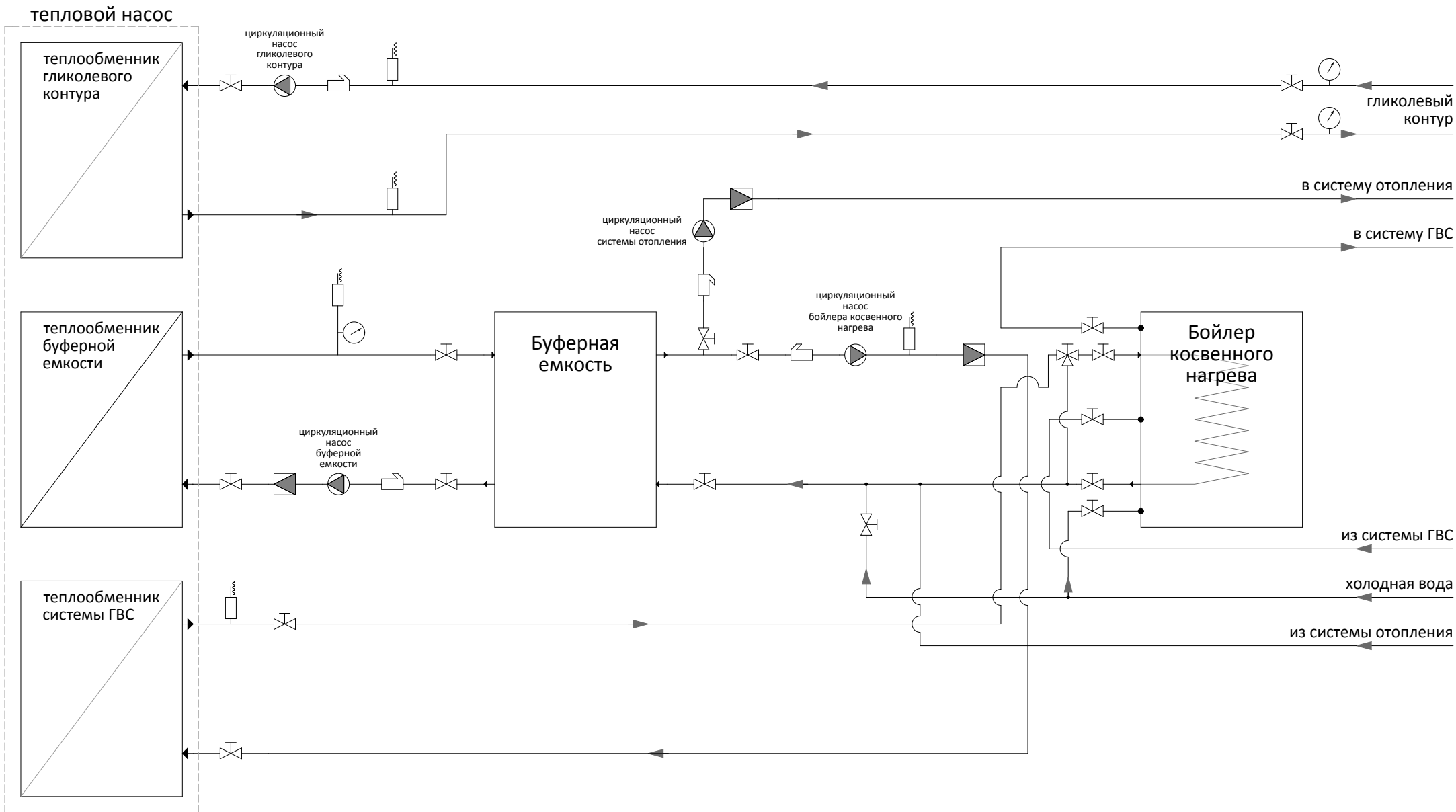
Схема подключения теплового насоса к системе отопления и ГВС
